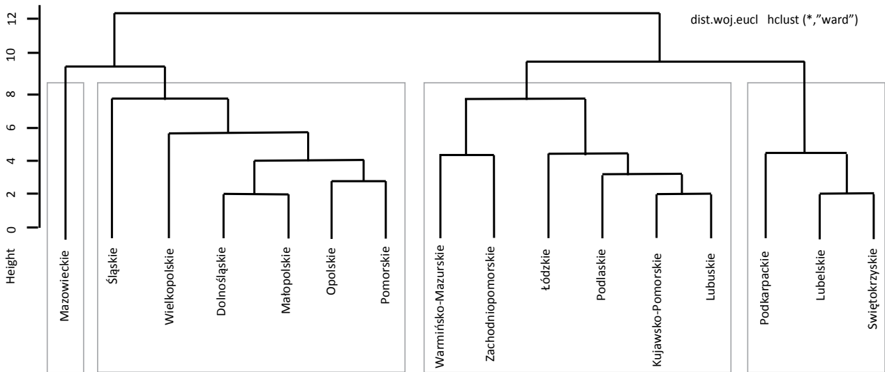
Rysunek 7. Metoda Warda, odległość euklidesowa
